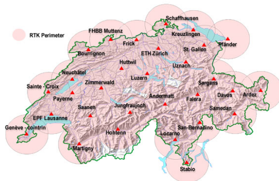
Figura 5: Red VRS en Suiza con GPSNet de Trimble
