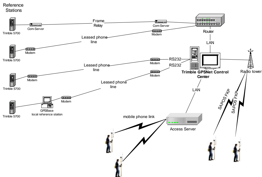
Figura 8: Esquema de conexiones con servidor de acceso
