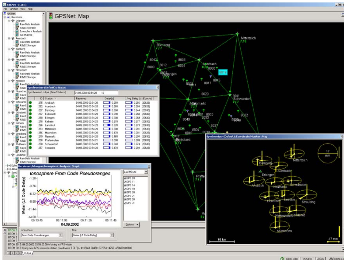
Figura 9: GPSNet gestionando una red VRS mostrando posiciones de los “rovers” conectados, retardos en las señales desde las estaciones, actividad ionosférica y control de coordenadas de las estaciones.
